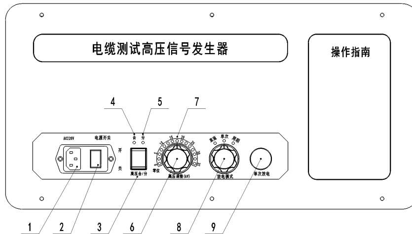
图 2-2-1 控制面板
