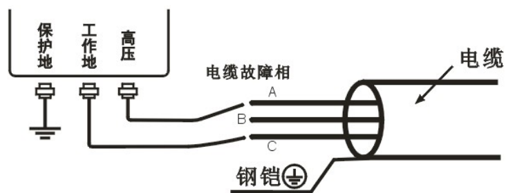
3-1-2 相间故障接线示意图
