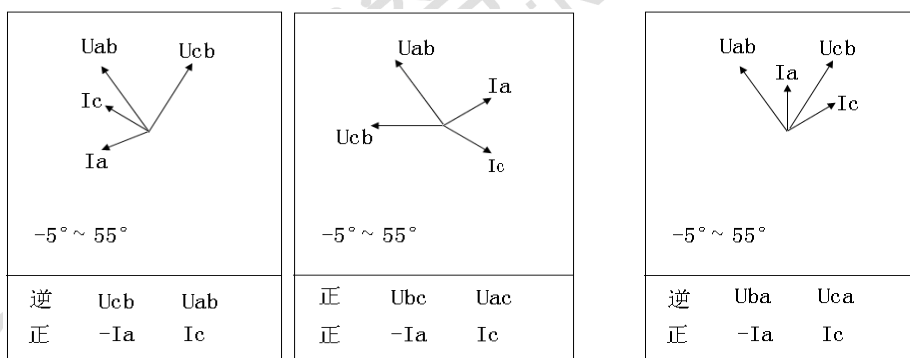
A、C相电压接反
