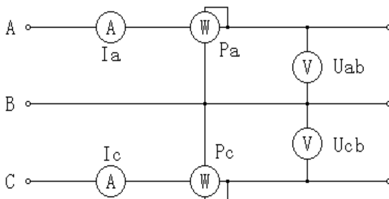
图十九、三相三线计量原理图
