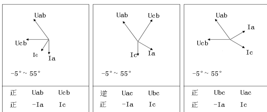
A、B、C三相电压接线正确
