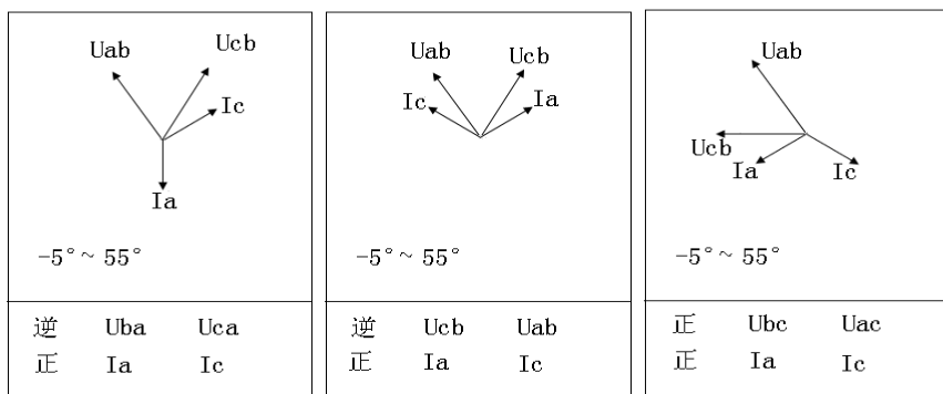
A、B相电压接错
