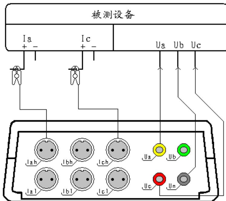
图三十、三线计量矢量测试
